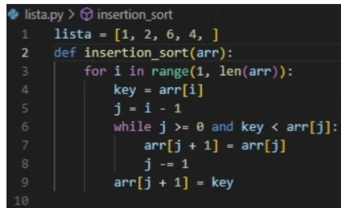
Figura 4.7: Tela de Implementação do P7
